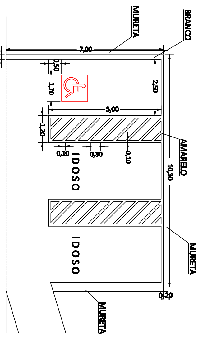
DETALHE ESTACIONAMENTO PCD ESCALA 1/100
